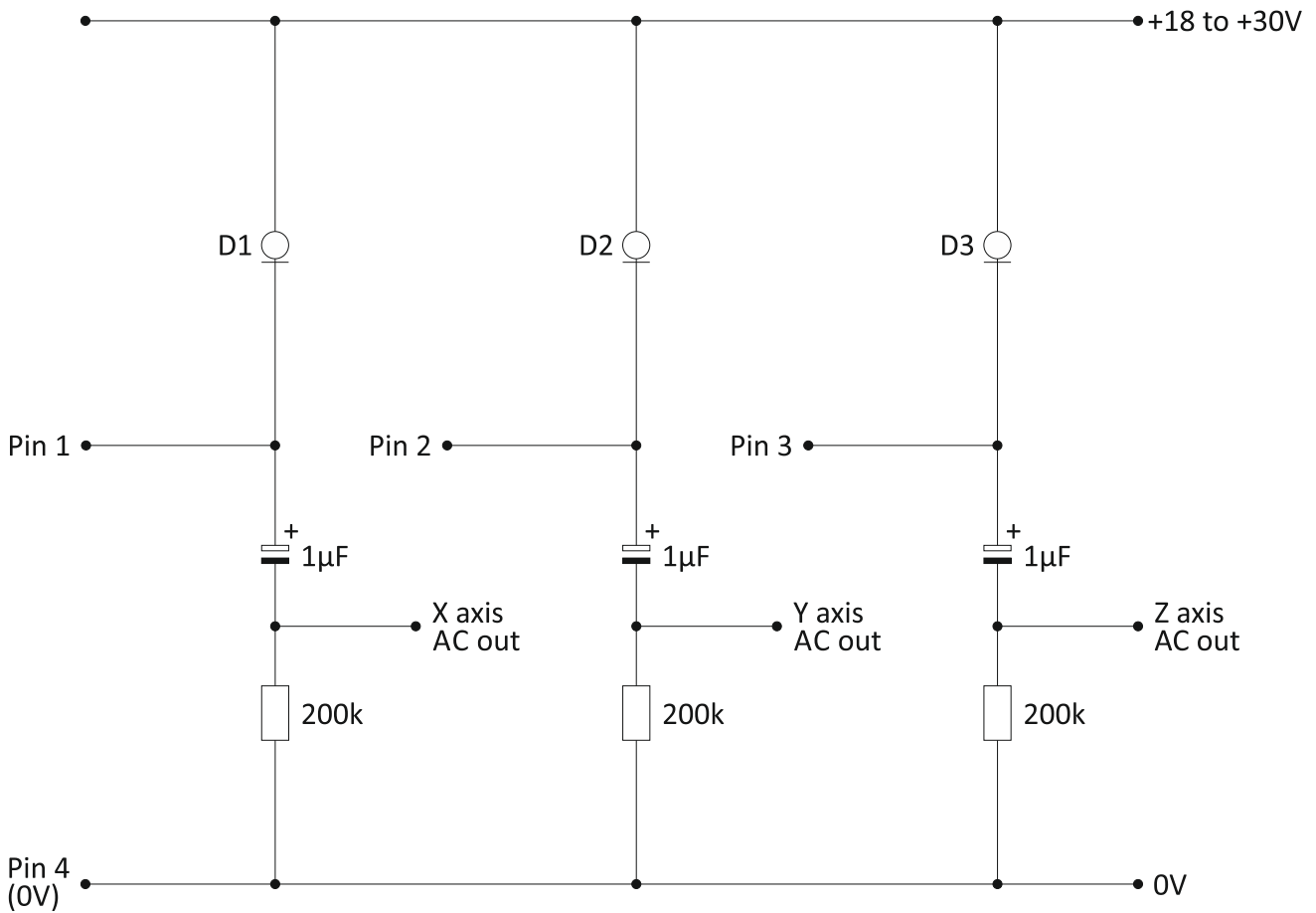
D1;D2;D3 Constant current diode (0.5-8.0mA)
